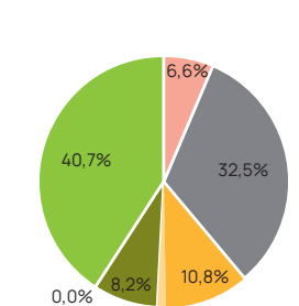
Energieträgermix Deutschland**
