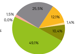
Energieträgermix Deutschland**
