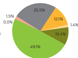
Energieträgermix Deutschland**
