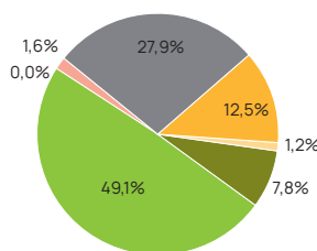
Verbleibender Energieträgermix*
